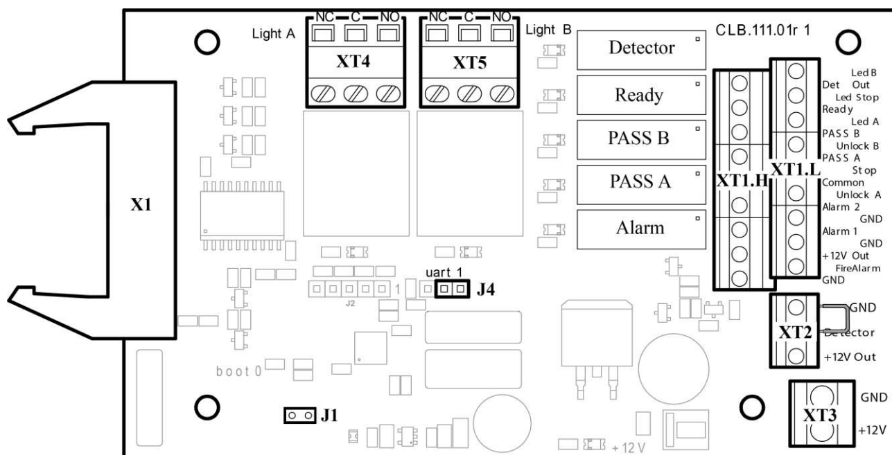
Рисунок 5. Внешний вид платы CLB
